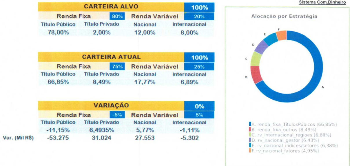
Figura 2 Alocação Alvo
